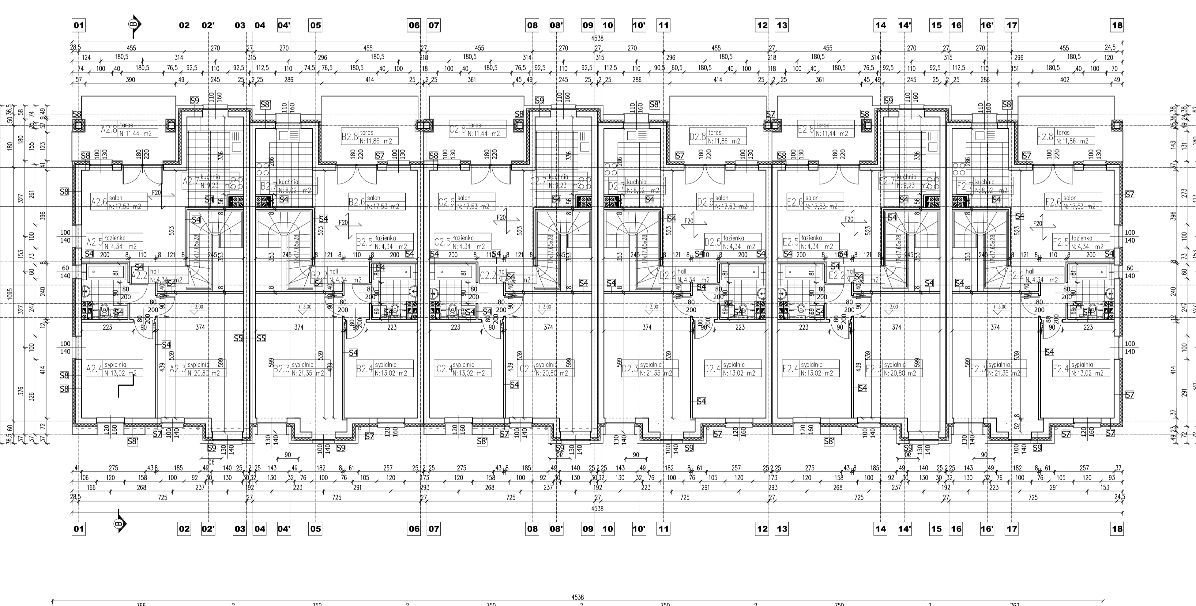
RZUT PIĘTAR
