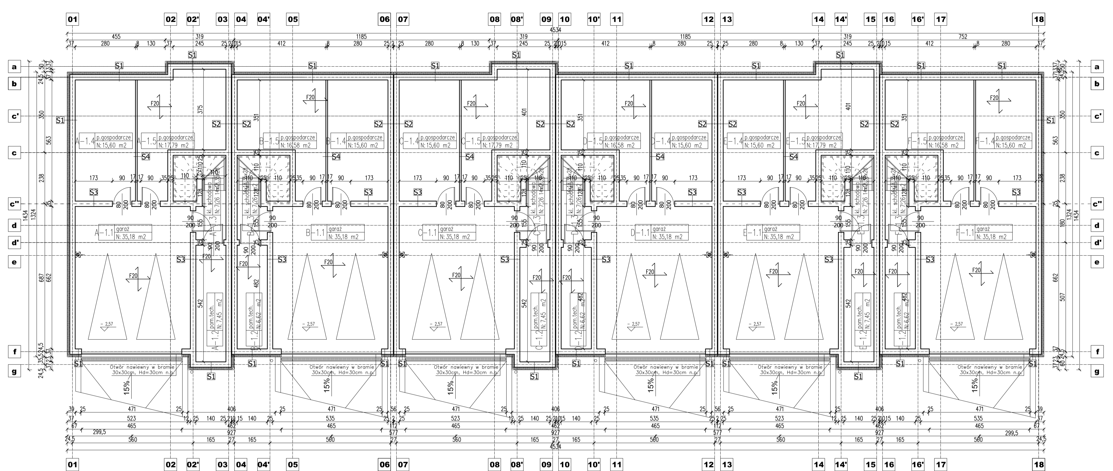
RZUT PIWNIC
